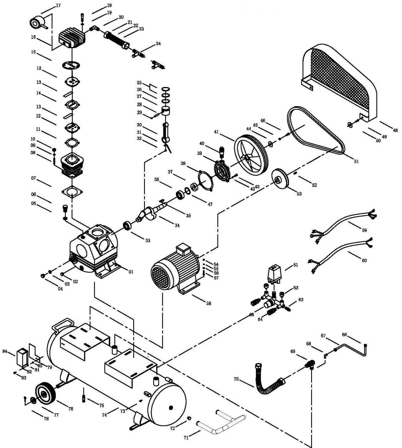
Рисунок 2. TORNADO 140
